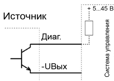
Рисунок 12 – Пример подключения вывода «Диаг.»
