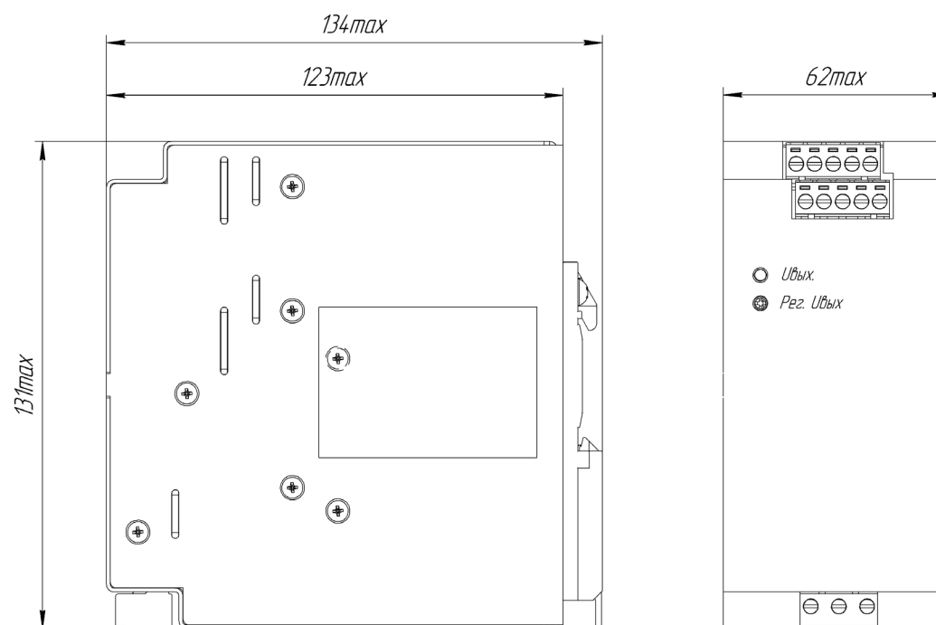
Рисунок Г.3 - Габаритные размеры Источников КАН-Д240 и КАН-Д480
