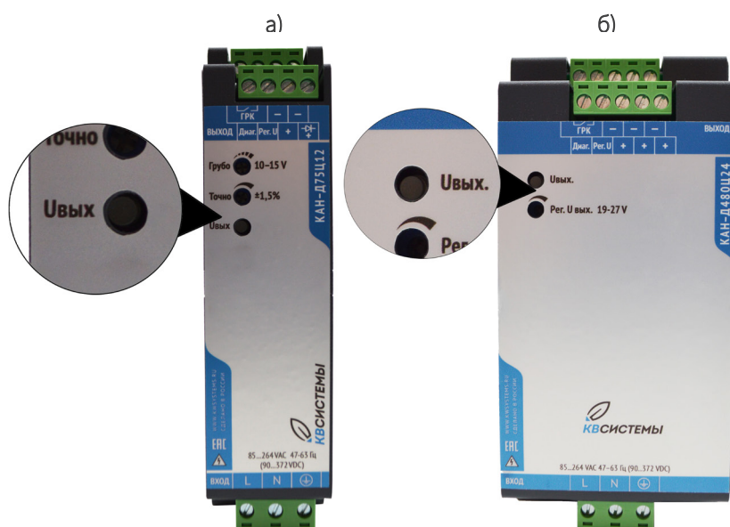
Рисунок 15 - Индикатор состояния выходного напряжения Источника: а) КАН-Д75; б) КАН-Д120, КАН-Д240 и КАН-Д480
