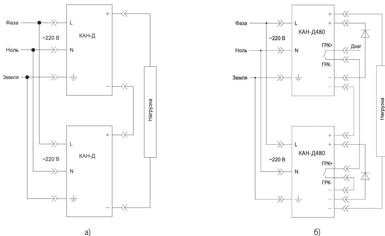
Рисунок 22 – Последовательное включение Источников: а) КАН-Д75, КАН-Д120, КАН-Д240; б) КАН-Д480
