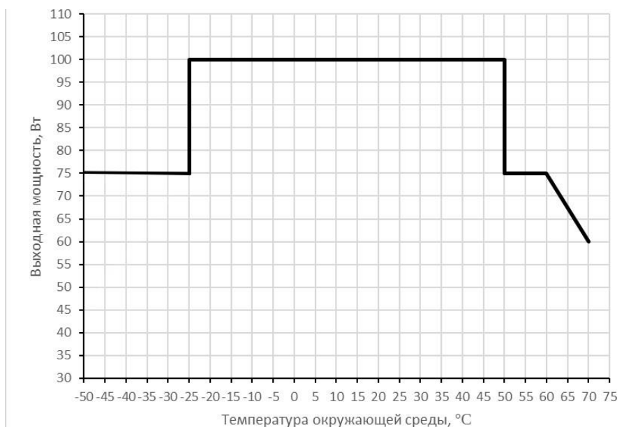
Рисунок А.1 - График зависимости максимальной выходной мощности от температуры окружающей среды для КАН-Д75: а) исполнения «Н»; б) исполнения «П»
