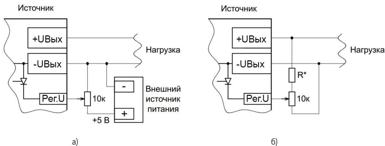
Рисунок 13 – Регулировка выходного напряжения с помощью вывода «Per.U» при подключении: а) к внешнему источнику питания +5 В; б) к выходу Источника.
